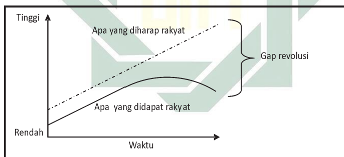
Gambar 4 Kurva Teori Revolusi
