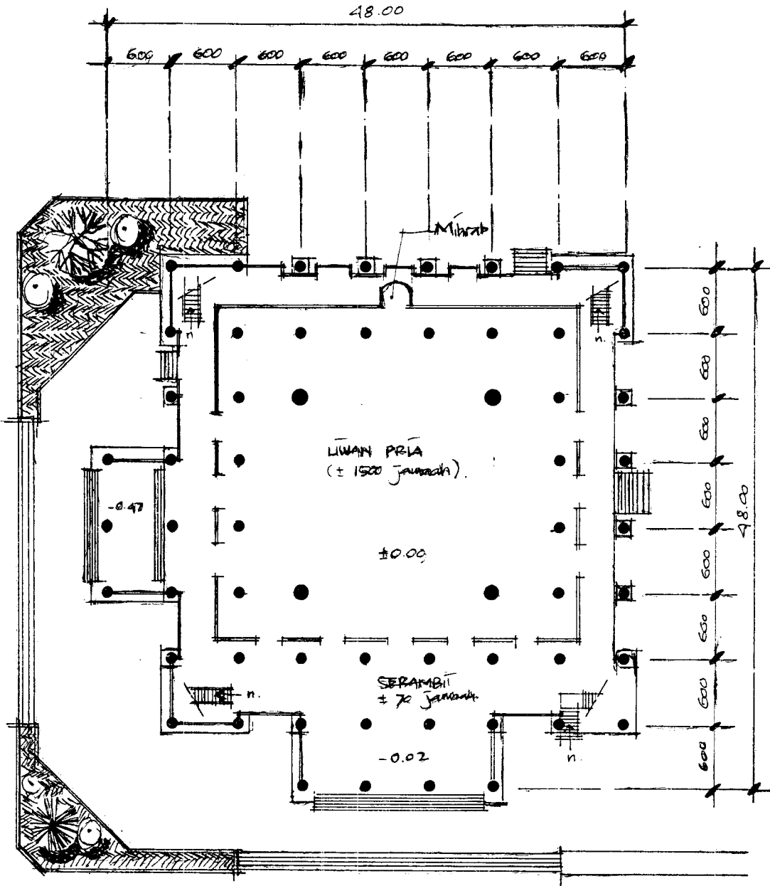
DENAH LANTAI BAWAH
